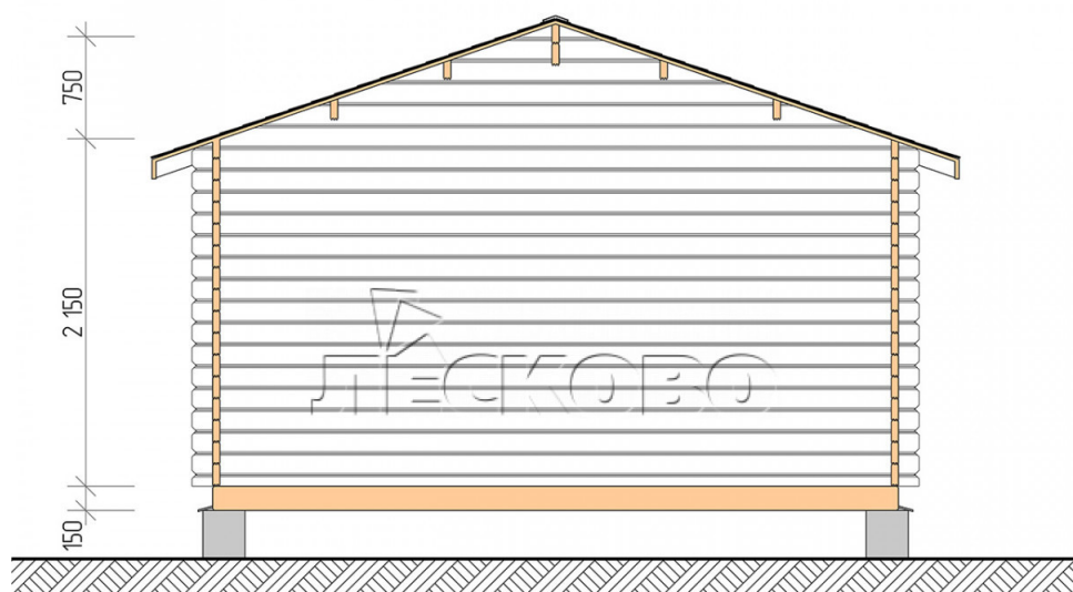
Разрез
