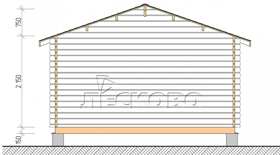
Разрез
