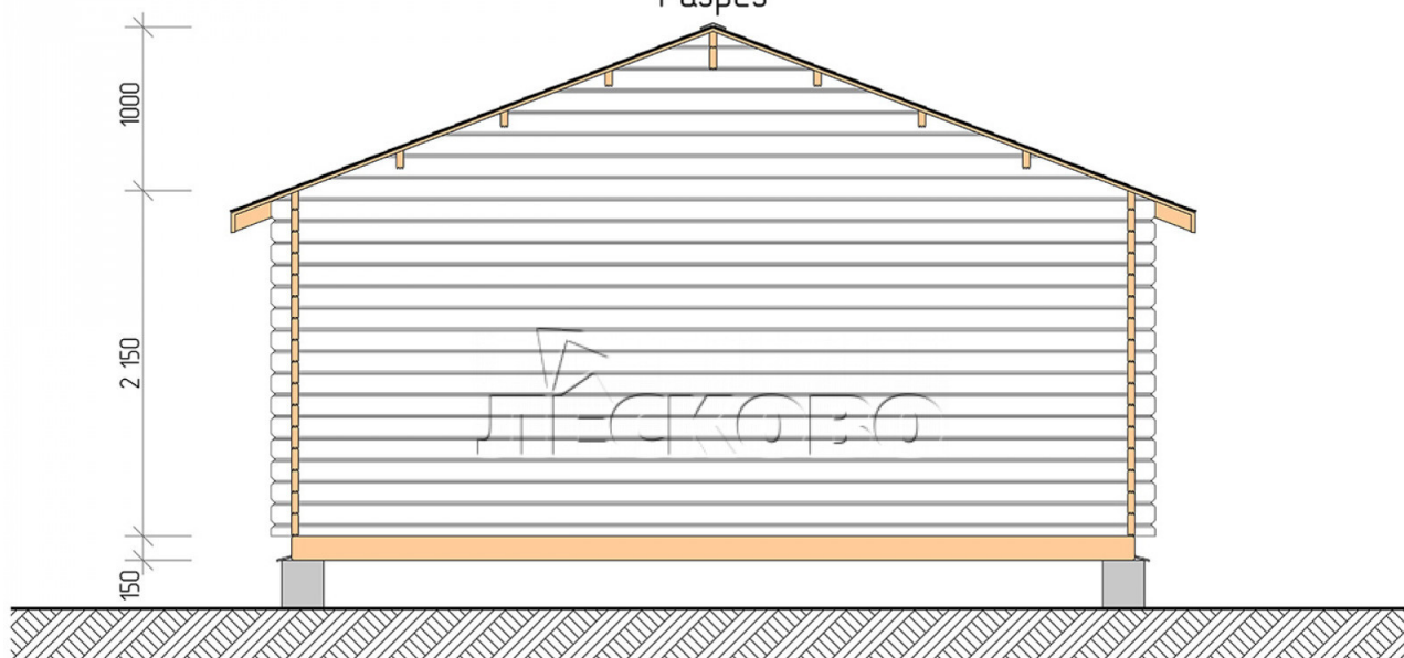
Разрез
